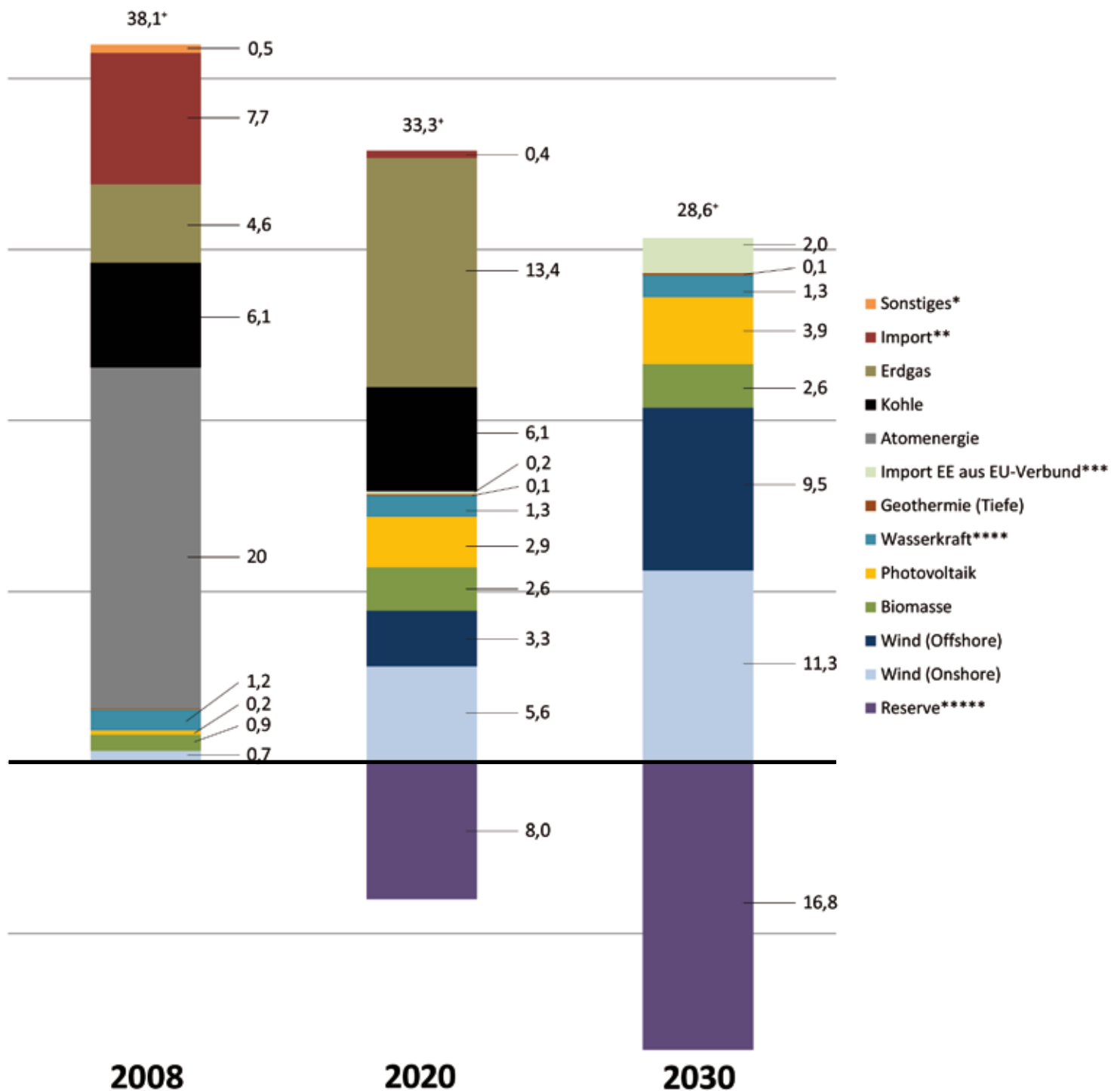
ABBILDUNG 1: ZUKUNFTSENERGIE FÜR HESSEN - ENTWICKLUNG DES STROMMIX BIS 2030 IN TWh/a.
